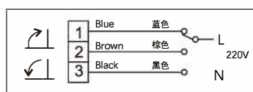
三线开关控制(三线双控)
