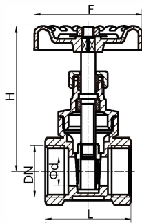
WG91: 黄铜
