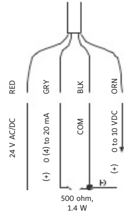
图5: 24V模拟控制 - 0 (4)-20 mA
